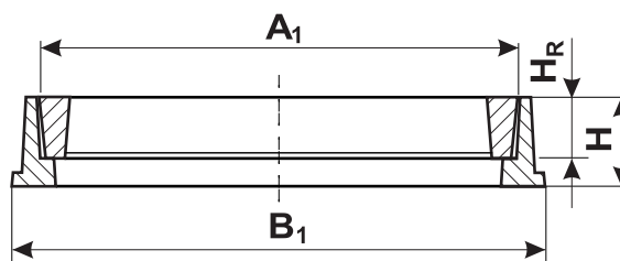
Presjek A-A:
