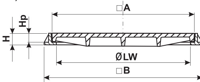
Presjek A-A:
